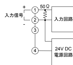
アイソレータとしてご使用の場合
