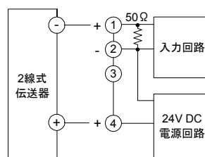
ディストリビュータとしてご使用の場合
