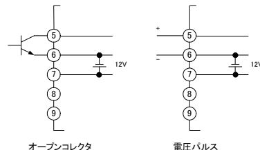
オープンコレクタ
