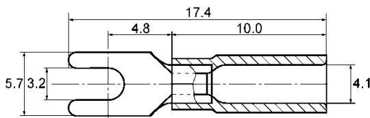
Y形圧着端子外形図
