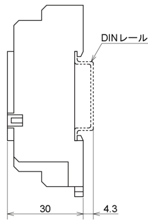
11P ソケット(SGFW)
