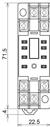
8P ソケット(SGF, SGFL)
