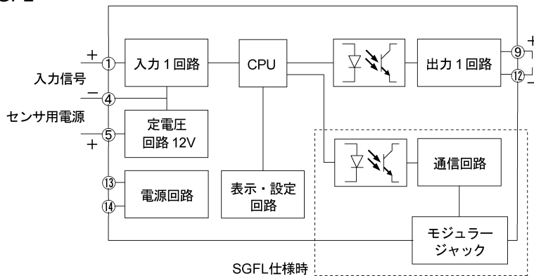
SGFL仕様時 (図4.2-1)
