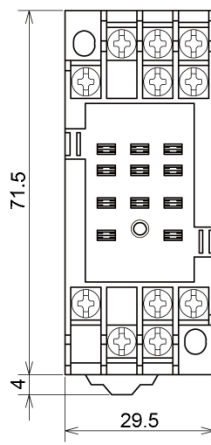
11P ソケット(SGFW)
