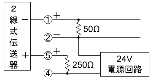
(図4.3-2 2出力(入力抵抗約300Ω))
