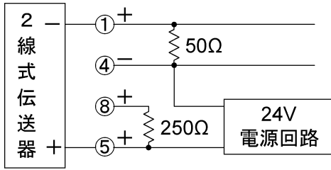
(図4.3-3 1出力(入力抵抗約50Ω))
