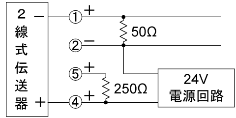
(図4.3-4 2出力(入力抵抗約50Ω))
