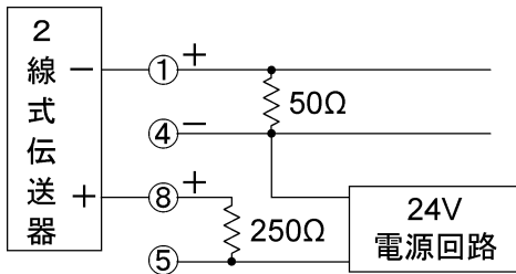
(図4.3-1 1出力(入力抵抗約300Ω))
